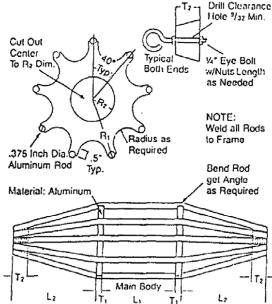
Go/No Go Mandrel
